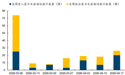
图表1：本周通过霍尔木兹海峡船只数量进一步回升
