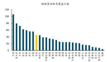
图表18：全球主要国家陆地原油储备对每日消耗的平均覆盖天数约为 45 天
