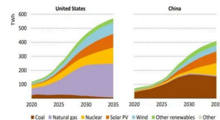
图表16：国际能源署预测，至 2035 年中美数据中心耗电总量将从当前的约 300TWh 增长至约 1000TWh
